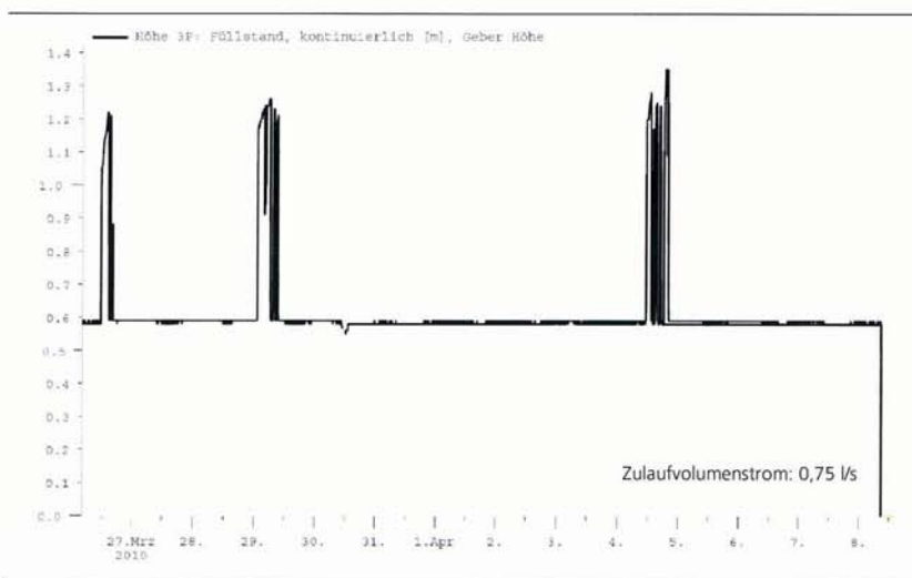
Bild 15 Füllstandsmessung Überlaufrohr 25.03. - 06.04.2010 vor der Filterspülung
