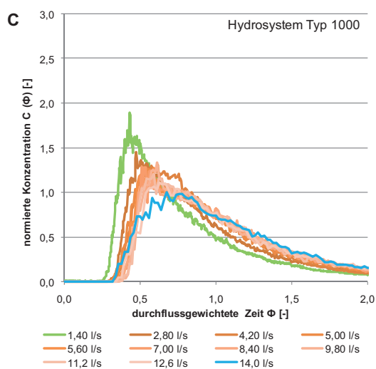
Abbildung 3-1: Verweilzeitdichteverteilung
