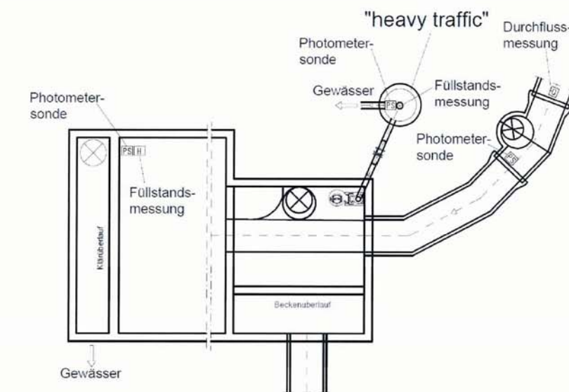
Bild 3 Einbauorte der Messtechnik auf der Versuchsanlage „Kulloch“
