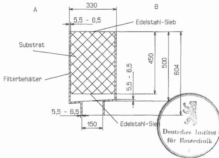
Schnitt A-B
