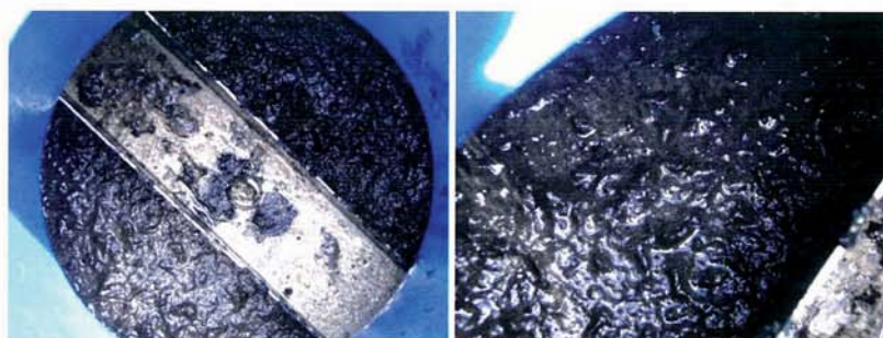
Bild 14 Filtererschöpfung durch Ausbildung Filterkuchen auf dem Zulaufsieb
