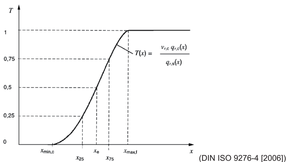
Abbildung 2-4: Trenngradkurve
