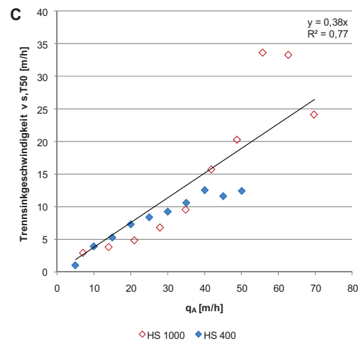
Abbildung 3-14: Reinigungsleistung der Anlage
